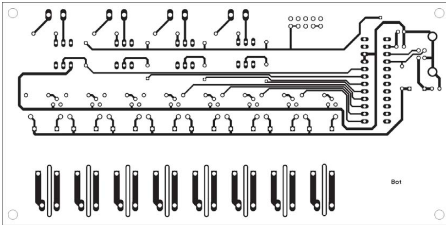
Bild 3: Leiterführung auf der Lötseite; die 152 mm × 76 mm große Platine hat zwischen den Relaiskontaktpins und Schraubklemmen geätzte Schlitze. Maßstab 1:1,25
