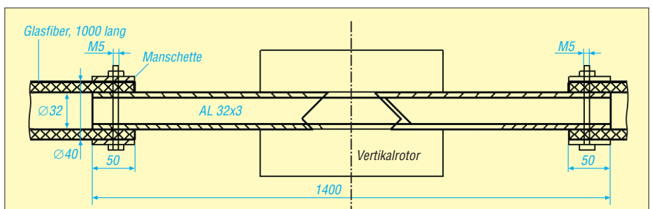
Bild 2: Die Konstruktion des Querrohrs als zerlegbare „Extra-leicht-Version“. Die bei relativ leichten Glasfaserrohren von 40 mm Durchmesser durch den Wind recht schnell verursachten Dreherschwingungen werden durch Verwendung eines Aluminiumrohrs außerhalb der kritischen Antennenzonen vermieden.
