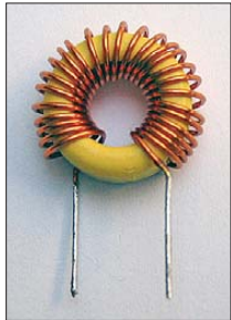
Bild 11: Bewicklung der Ringkerne für die Spulen L1 bis L4 des Preselektors am Beispiel von L3
