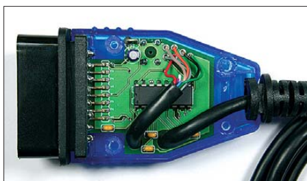
Bild 12: Oberseite des geöffneten OBD2-Steckers; der MAX3232 ist mit gekürzten Anschlüssen einzulöten.
