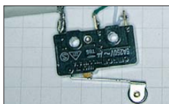
Bild 2: Ansicht des verdrahteten Mikroschalters für den Impulsgeber
