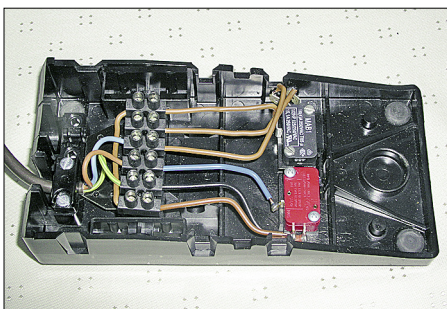
Bild 7: Damit die Hände zum Führen des aufzuwickelnden Drahtes frei sind, sollte ein entsprechend verdrahteter Fußschalter zum Einsatz kommen. Fotos: OE1MSA
