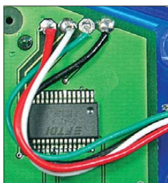
Bild 7: Anschluss des Kabels der USB- Schnittstelle; +USB → rot, D+ → weiß, D- → grün, -USB → schwarz
