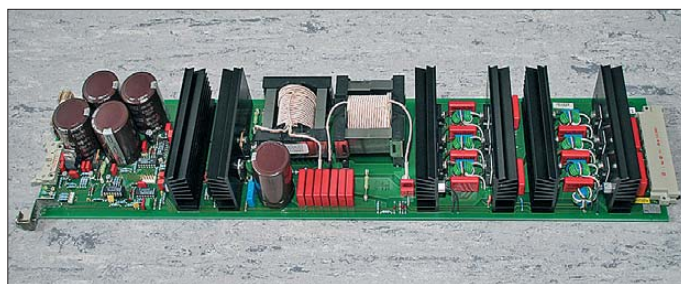
Bild 3: Leistungsmodul der Endstufe
