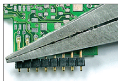
Bild 10: Mit einer Zange und sanfter Ge- walt lässt sich der Isolierkörper von den Stiften schieben.
