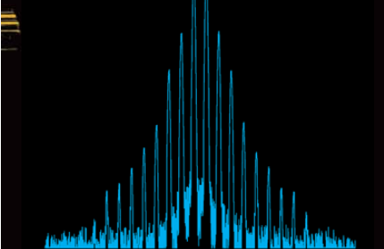
IM-Verhalten einer HLV 1500 bei 1000 W PEP
