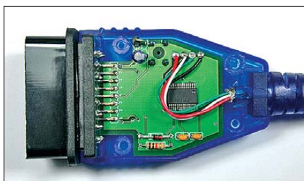
Bild 14: Oberseite des geöffneten OBD2-Steckers; der FT232RL ist in der USB-Variante bereits bestückt. Fotos: Stange, Reuss
