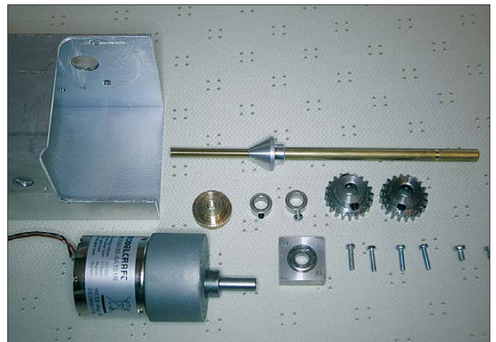
Bild 3: Für die Mechanik kommen nur Standardbauteile zum Einsatz: oben das bearbeitete Aluminiumprofil, die Messingspindel mit Aluminiumdrehteil, in der mittleren Reihe Rändelmutter, Abstandsringe und Zahnräder, in der unteren Reihe Getriebemotor, Kugellager mit Lagerbock und diverse Schrauben.
