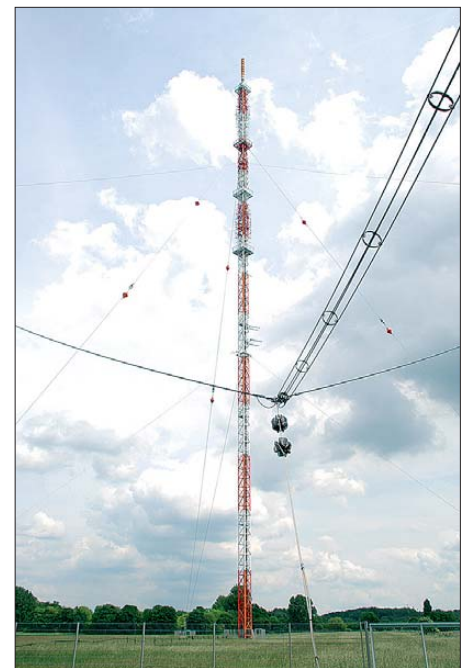
Bild 6: Reusenförmige Speiseleitung, rechts und links die Drähte der rauteförmigen Antenne Fotos: DL6AKC
