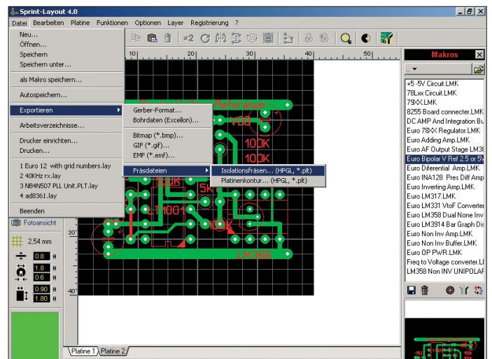
Bild 12: Sprint-Layout unterstützt u. a. den Betrieb eines Fräseplotters.
