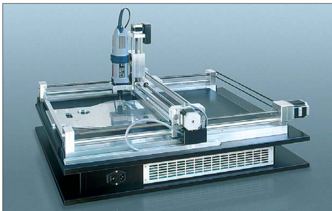
Bild 11: Fräseplotter von Haase Computer-technik [7]
