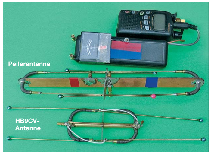
Bild 6: Transportfertig gefaltete Antennen, Peilerbaugruppe mit Stromversorgung und Anzeigeinstrument sowie Empfänger; die gesamte Ausrüstung passt in einen kleinen Stoffbeutel. Fotos: DL9SU
