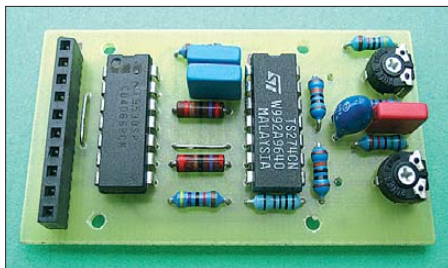
Bild 4: Fertige bestückte Platine; es werden ausschließlich bedrahtete Bauelemente verwendet.
