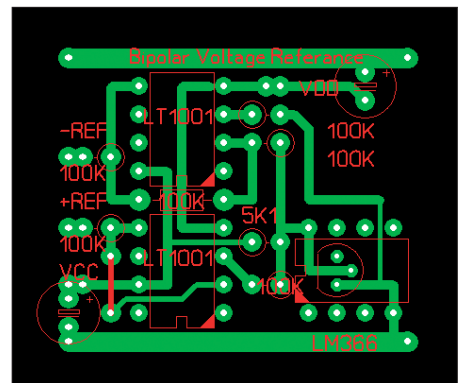
Bild 7: Beispiel einer Funktionsbaugruppe: bipolare Referenzspannungsquelle mit LM386
