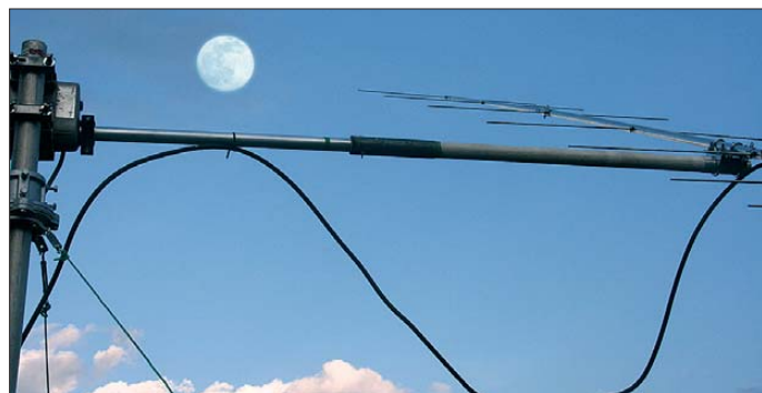
Bild 3: Der Querträger mit montierten Antennen in Aktion, genau auf das Ziel ausgerichtet
