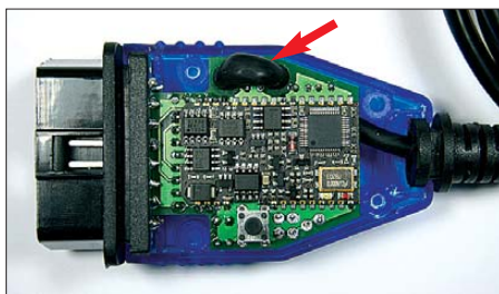
Bild 11: Platinenunterseite mit dem DXM-Modul in der RS232-Variante, erkennbar am durchgefädelten Kabel
