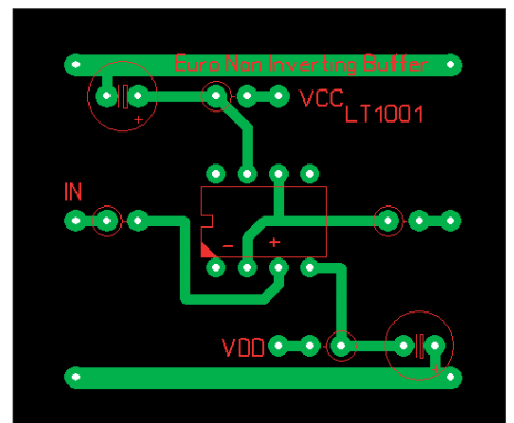
Bild 10: Beispiel einer Funktionsbaugruppe: nichtinvertierender Puffer mit LT1001
