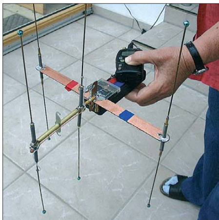
Bild 1: Vollständiger Aufbau des Phasenpeilers einschließlich Antennen
