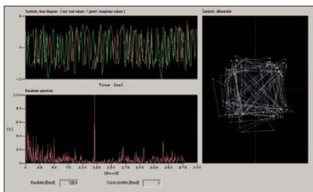
Das System AT3004D, 12 x 120 Bd, hier: QPSK mit Piloton, 2600 Hz breit (W61-Classifizierung-Analyse)
