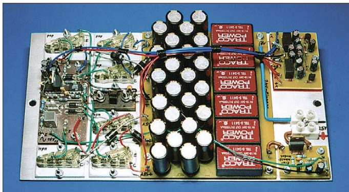
Bild 1: Der Prototyp des Verstärkermoduls besteht aus mehreren Einzelplatten auf einer Grundplatte: v. l. n. r. Treiber mit vergossenen Endstufentransistoren, Hauptspannungserzeugung, Spannungserzeugung für Treiber und Einschaltmodul.
